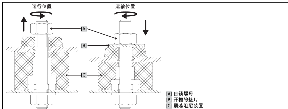
运输保护装置的示意 图型号 B
