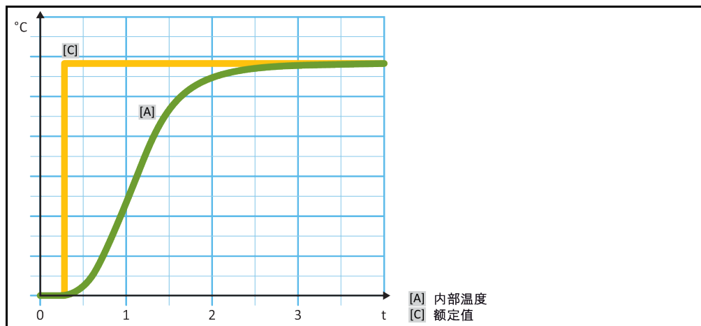
内部、非周期性温度控制
