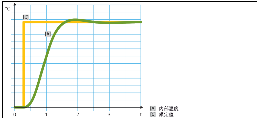
内部动态温度调节，可能有温度过冲
